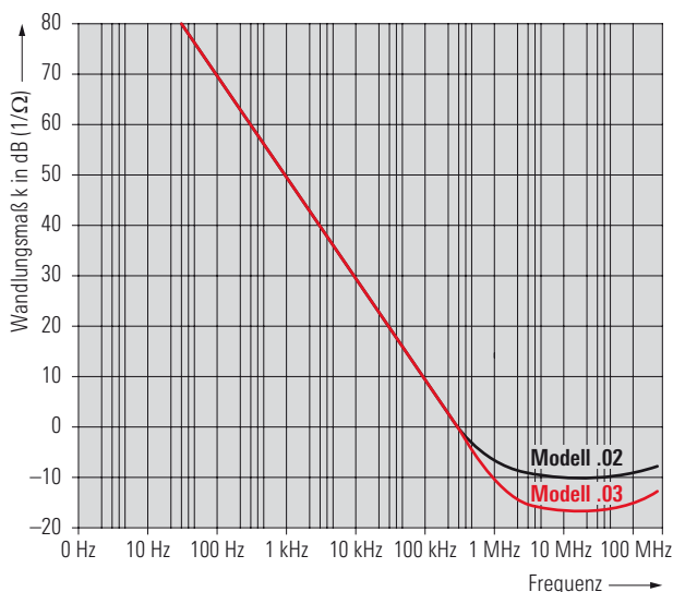
Wandlungsmaß k der zwei Modelle des Stromwandlers R&S®EZ-17
